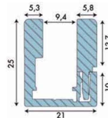
Plan de coupe Profil à parecloses
